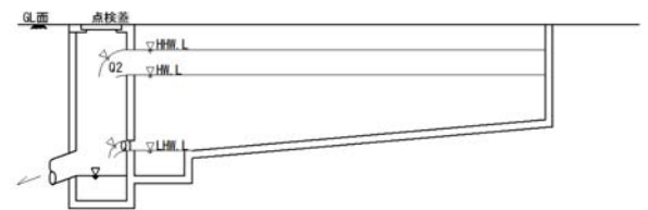
図-3 側溝を利用した貯留施設のイメージ図
