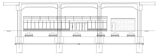
図-2 高架標準断面図
