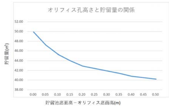
図-11 オリフィス高と貯留量の関係
