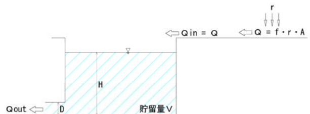
図-8 自然放流式貯留模式図
